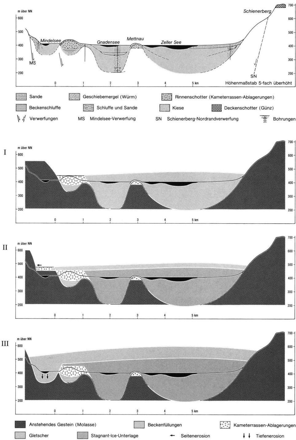
Abb. 20: Querprofil über den zentralen Untersee und seine Flanken (nach SCHREINER 1968, oben) und die Deutung des Nebeneinanders von Kamterrassen und übertieften Rinnen (darunter). Zur Lage des Profils vgl. Abb. 19. Näheres im Text. Fig. 20: Cross-section of the central Untersee basin and its flanks (after SCHREINER 1968, above) and the interpretation of the side-by-side occurrence of kame-terraces and overdeepened channels (underneath). For location of the cross-section see fig. 19, for details see text.
