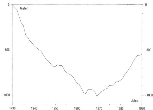
Abb. 12: Schwankungen des Zungenendes des Sólheimajökull – eines Fußgletschers des Myrdalsjökull – seit 1930 (nach NORDDAHL 1994, umgezeichnet).
