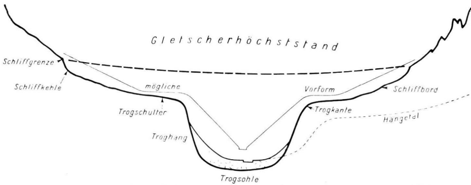
Schematischer Querschnitt eines alpinen Trogtals mit Trogschultern; Abb. 176 in Anlehnung an Louis/1952.
