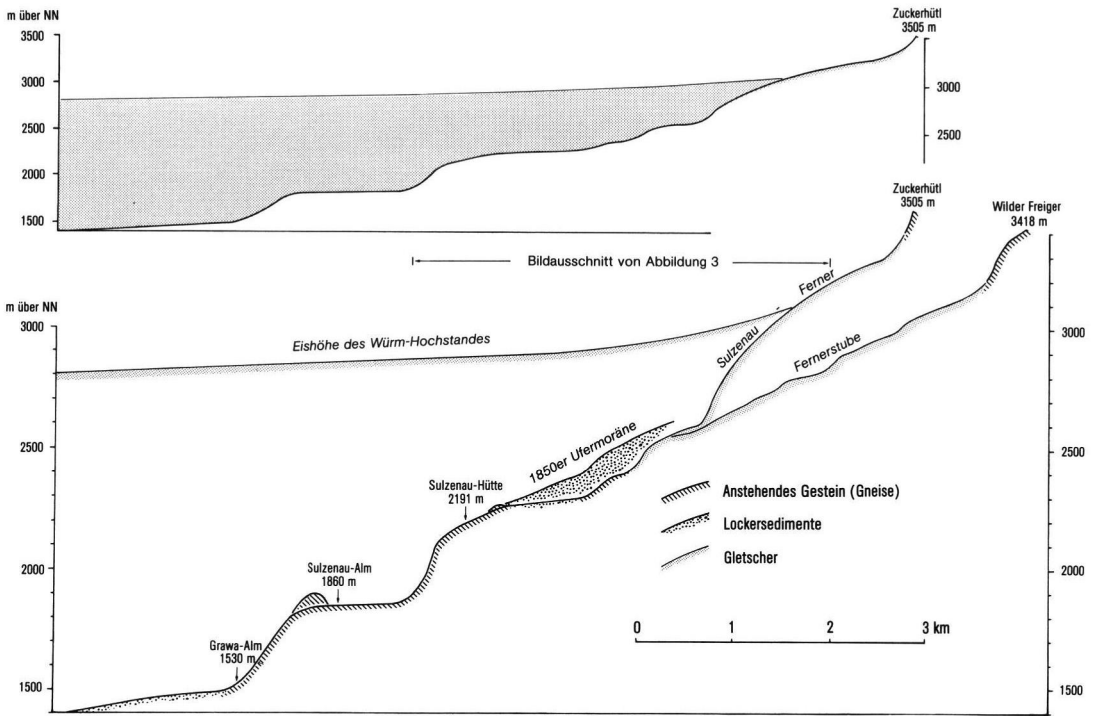
Abb. 4: Längsprofil der Sulzauferner-Talung, 2,5fach überhöht (unten) und nicht überhöht (oben). Obergrenze des Gletschers während des letztkaltzeitlichen Hochstandes in Anlehnung an VAN HUSEN (1987). Näheres im Text.
